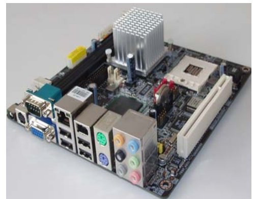
Pentium M Mini-ITX Board
