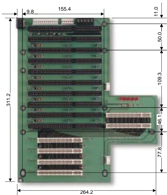
PBPI-14S2
