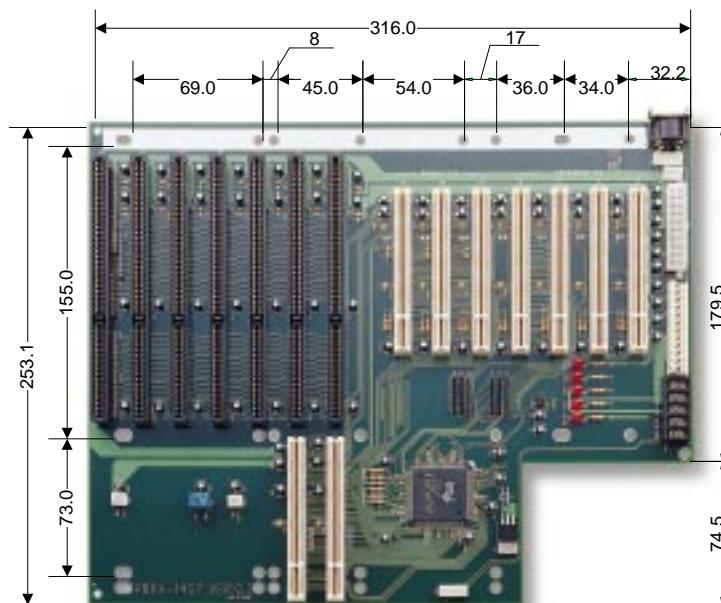
PBPX-14S7
